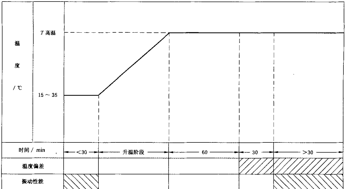
图 2 高温/振动综合检定程序图
